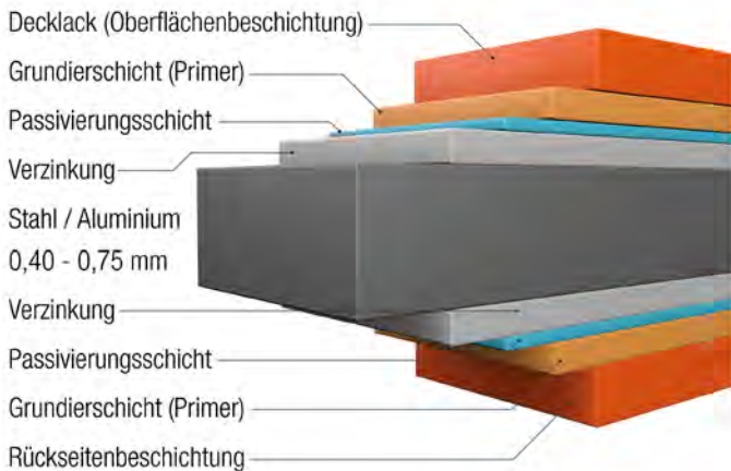
Beispiel: Beschichtungsaufbau
