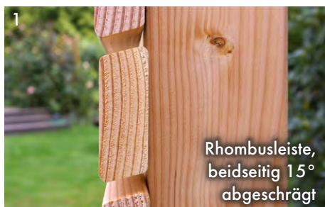
Rhombusleisten aus Fichte, kesseldruckimprägniert KDG grau Ausführung ohne Abdeckleiste
