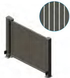
ST Paneel 110 Stabbreite 110 mm Stababstand ca. 30 mm
