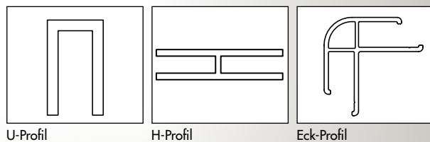
U-Profil
