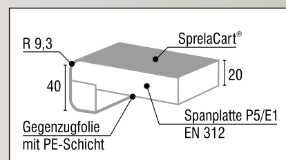
Profil 200 mit 40 mm Blende
