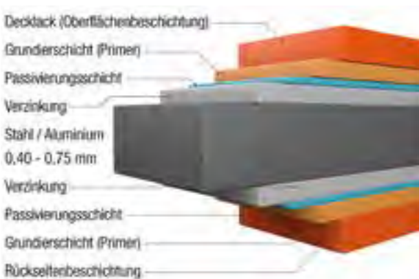
Beispiel: Beschichtungsaufbau
