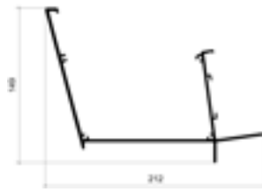
Standardrinne
