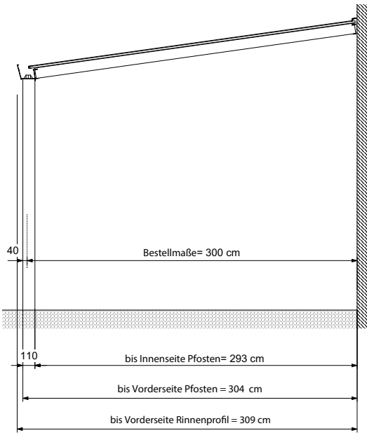
Standardrinne
