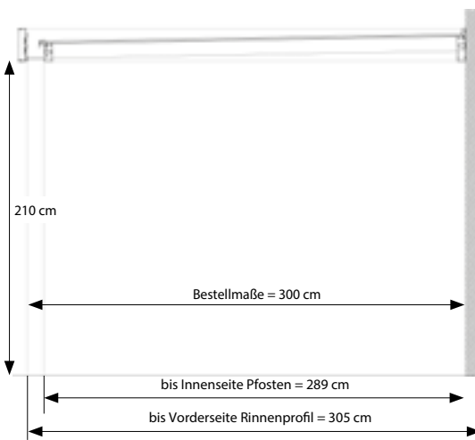
Standardrinne + Rinnenkappe
