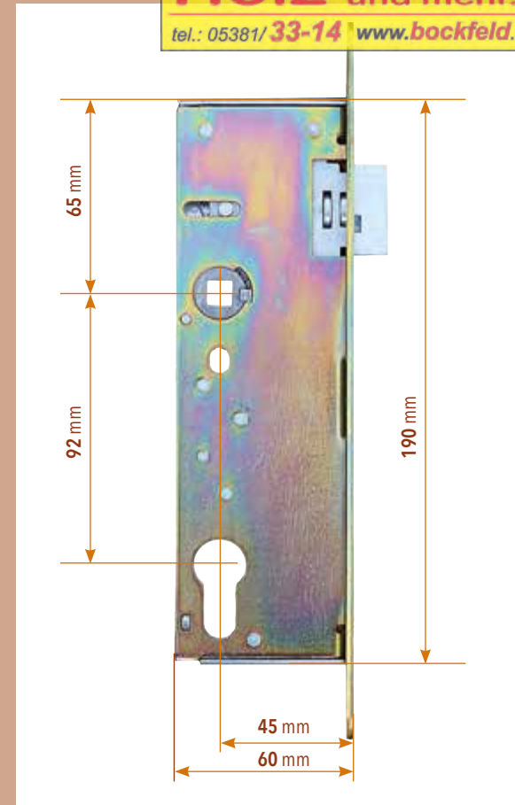
Einsteckschloss für Zauntore mit Ausfräsung
