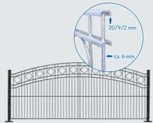
Dekor-U-Profilmatte mit Oberbogen und Ornament Karo
