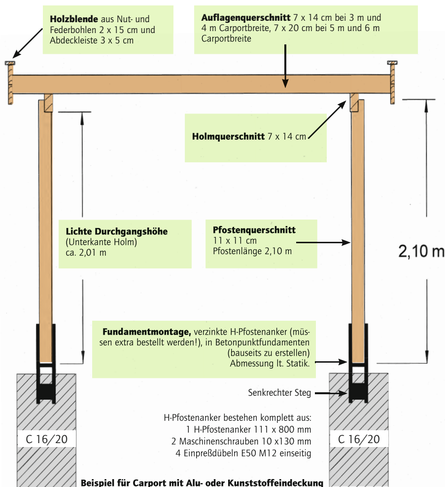
Beispiel für Carport mit Alu- oder Kunststoffeindeckung
