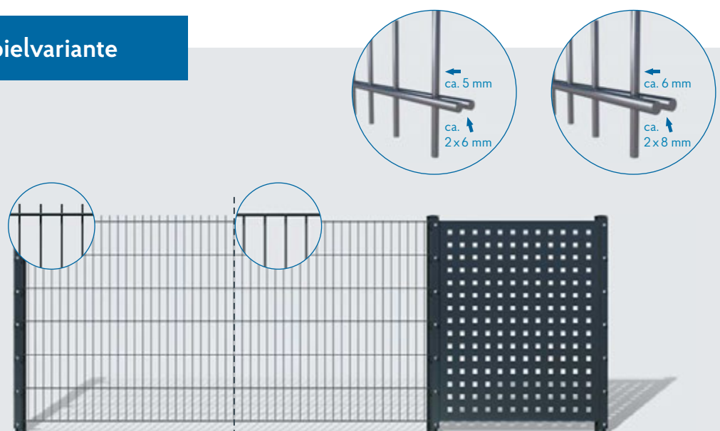
Doppelstabmatte mit Drahtüberstand / ohne Drahtüberstand / mit Loch-Designblech
