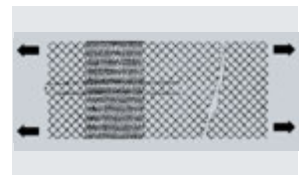
4. Matte zu einer Geflechtbahn auseinanderziehen.
