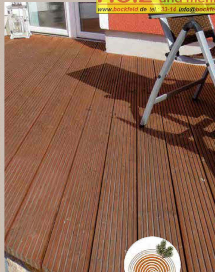
Kombi-Bodendiele aus Douglasie 2,7 cm stark, 14,6 cm breit, roh, beide Breitseiten unterschiedlich geriffelt.
