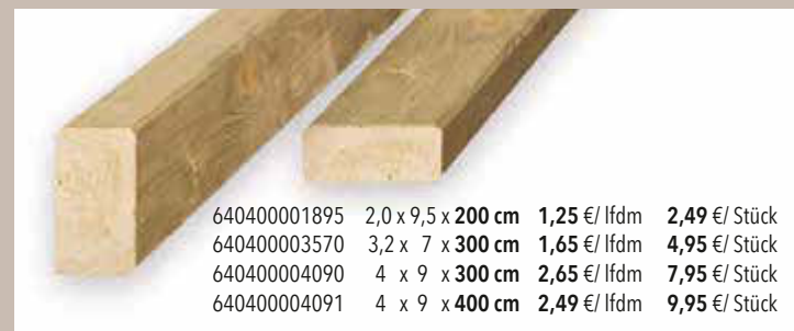
Konstruktionsholz aus Kiefer / Fichte glatt gehobelt und gefast, verschiedene Stärken und Längen, kesseldruckimprägniert
