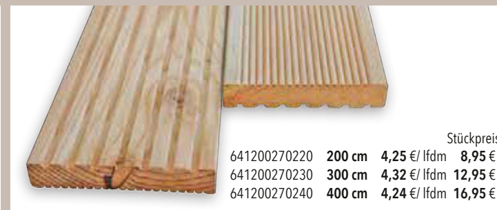
Kombi-Bodendiele aus Douglasie 2,7 cm stark, 14,6 cm breit, roh, beide Breitseiten unterschiedlich geriffelt.
