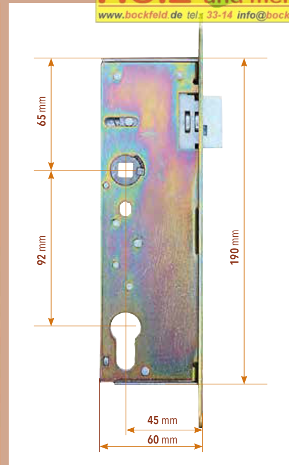
Einsteckschloss für Zauntore mit Ausfräsung
