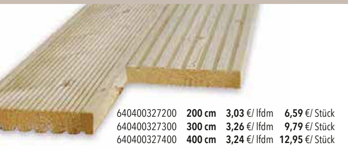
Kombi-Bodendiele aus Fichte 2,7 cm stark, 14,6 cm breit, kesseldruckimprägniert, beide Breitseiten unterschiedlich geriffelt.
